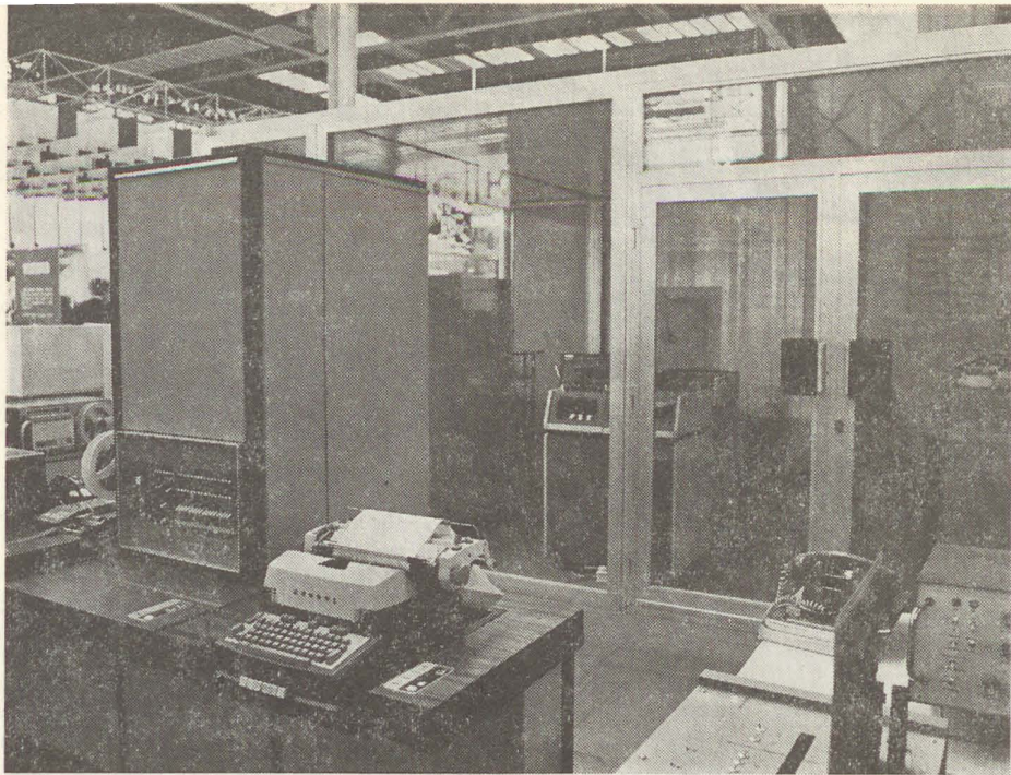
Az ESZ 1010 (R-10) magyar kissszámítógép sokperifériás konfigurációja. A háttérben, az üvegfalú kis klimatizált fülkében a kispéphez kapcsolt bolgár gyártású mágneslemezes tároló egységek.
