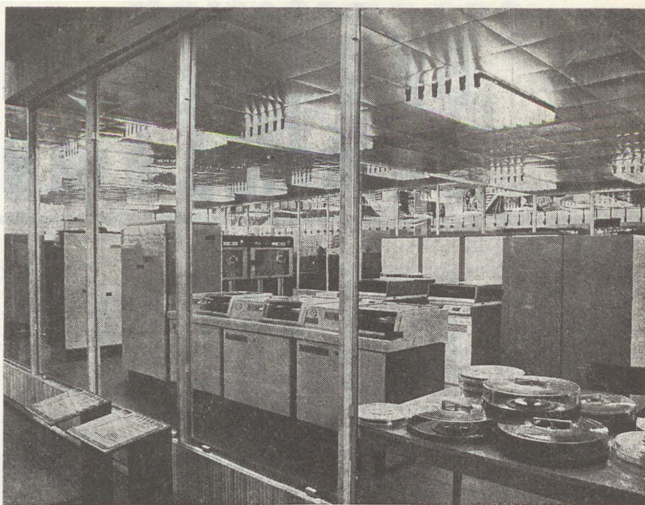
A központi standon, közös klimatizált teremben helyezték el az összes nagy gépkonfiguráció mágnesszalagos és mágnesszalagos egységeit.
