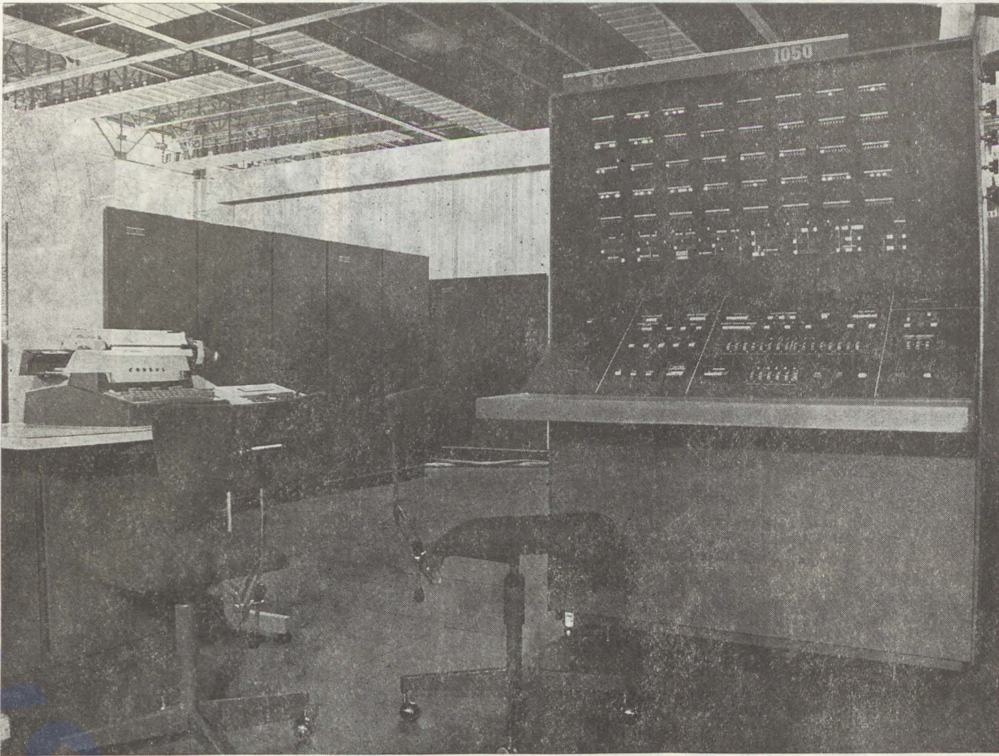
A kiállítás „sztárja”, a nyilvánosan első ízben itt bemutatott szovjet ESZ 1050 modell központi egysége.
