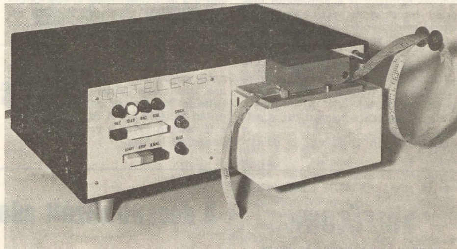
A Poznan-i Teletra cég UTD—114 Dateleks típusú berendezése 50 (200) baud sebességű adatátvitelre alkalmas.
