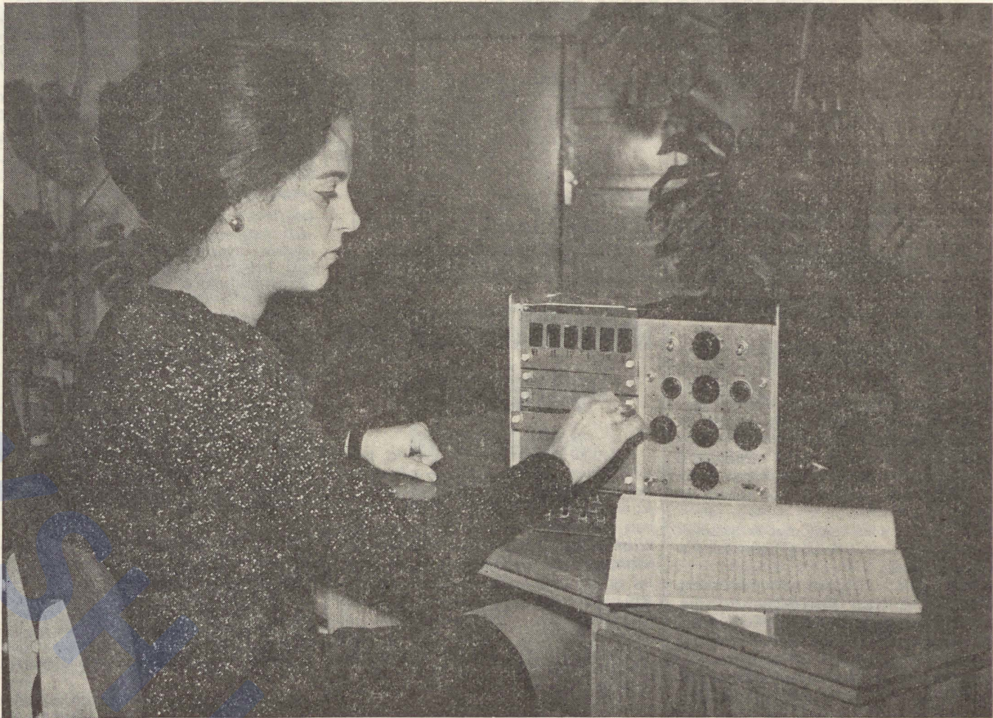
Képünkön hat sejtől álló sejtautomata látható működés közben. A készülékbe épített három ESZR kártya két sejtáramkört tartalmaz. A sajátos „számítógép” kicsiben szemlélteti a sejtautomaták alapelvét, azt, hogy műveletvégzés közben minden sejt egyidejűleg működhet.
