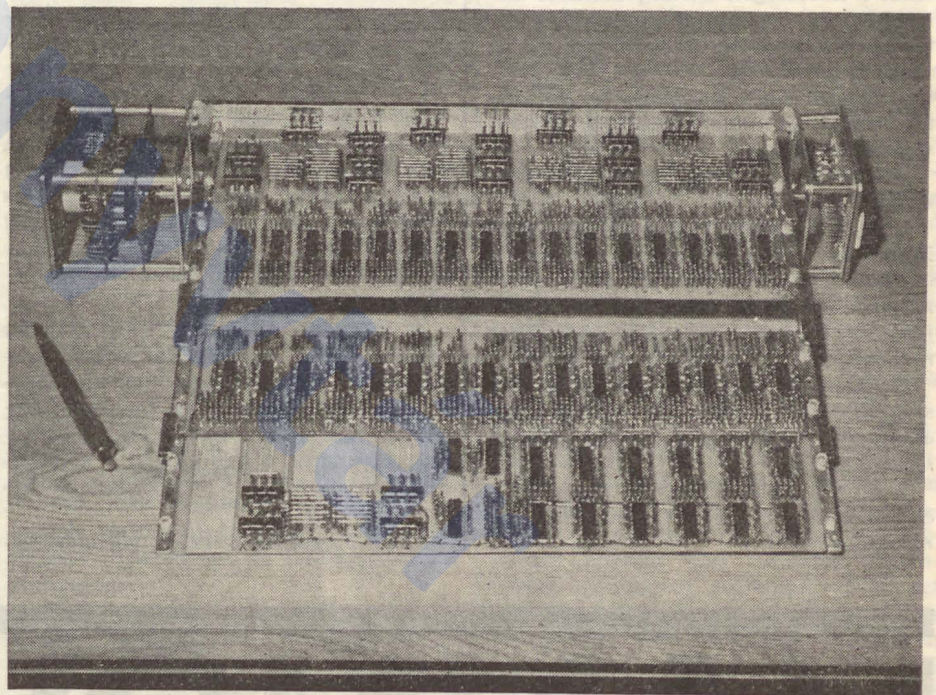
Egyetlen, számítástechnikailag univerzális sejt áramkörének képe. Az 1300 diódát tartalmazó „mindent tudó” sejt előnye, hogy elegendő számban alkalmazott, azonos áramkörökkel bármilyen számítógép-szerv kialakítható. A fejlesztés további feladata a sejt jelentős méretcsökkentésének megoldása.
