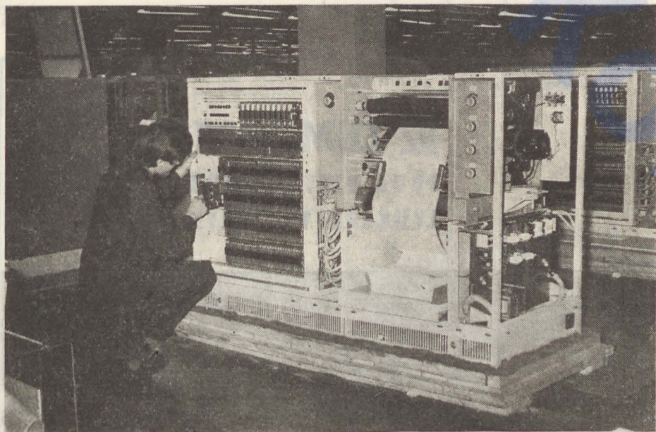
DW 21 típusú sornyomtatók a Blonie-i Finommechanikai Művek végbemérő részlegében.
